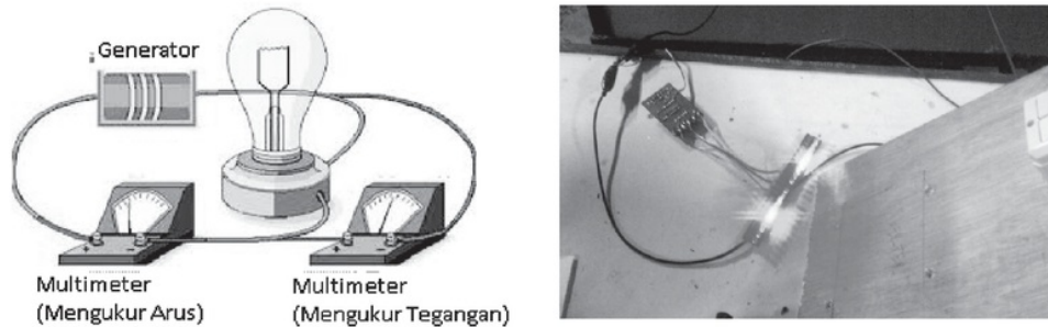
Gambar 5. Mekanisme pengambilan data tegangan dan arus listrik.
