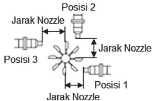
Gambar 3. Posisi dan jarak nozzle.
