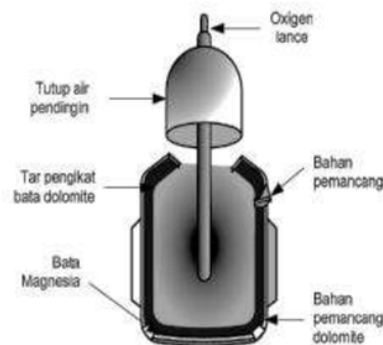
1 Gambar 2. 14 Proses Oksigen Pada Dapur Basa Untuk Pemurnian Besi Kasar (Akuan, 2014)
