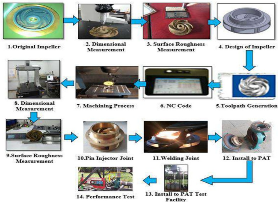
Gambar 5. 2 Alur Proses Pemesinan
