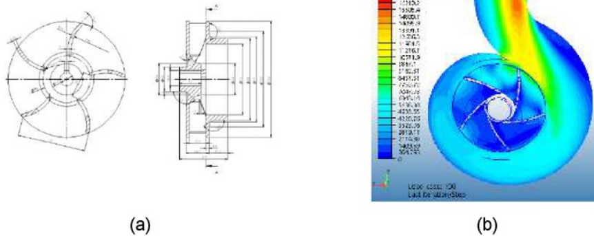
Gambar 5. 1 Modifikasi Impeller dengan 5 sudu
