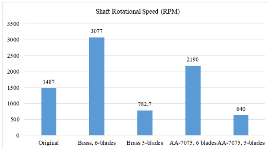
Gambar 5. 5 Kecepatan Putar Poros Pompa yang dihasilkan
