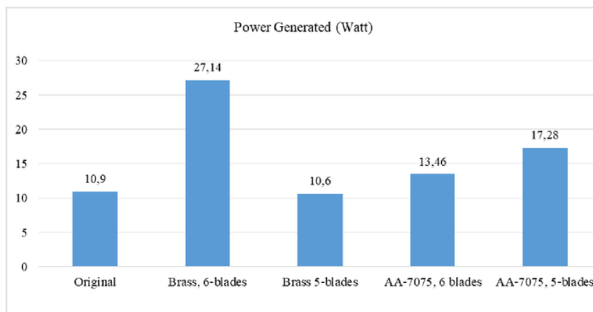
Gambar 5. 6 Energi listrik yang dihasilkan
