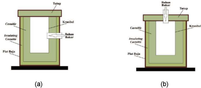
Gambar 5. 10 Variasi Posisi Burner (a) di samping, (b) di atas
