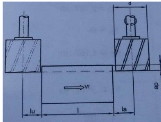
Gambar 2. 7 Gerakan face milling pada Mesin CNC [10]
