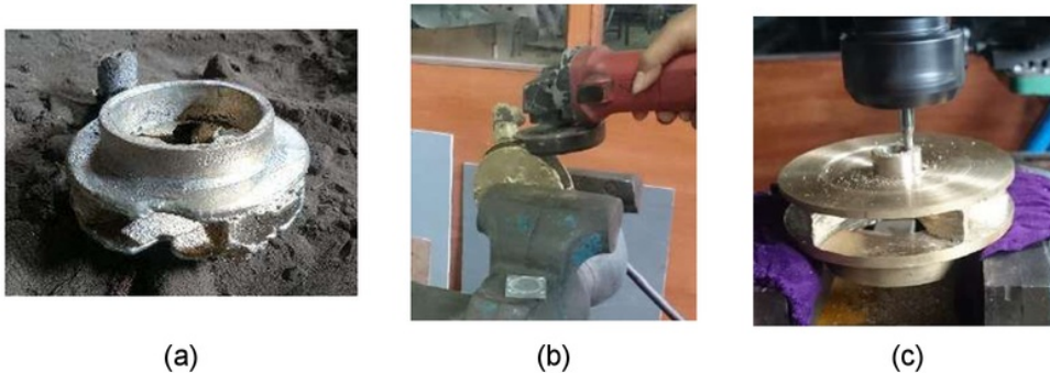
Gambar 5. 9 (a) Impeller Hasil Pengecoran, (b) Pemotongan Riser dengan Proses Grinding dan (c) Proses Finishing Milling
