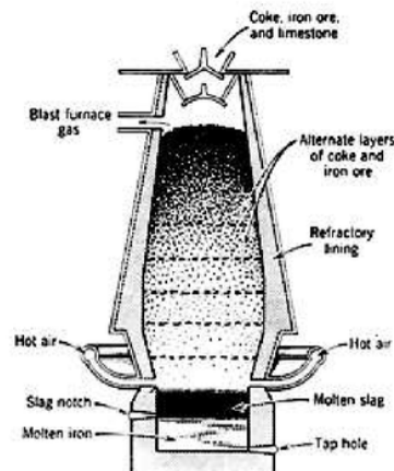
Gambar 2. 9 Tungku Kupola (Akuan, 2014)
