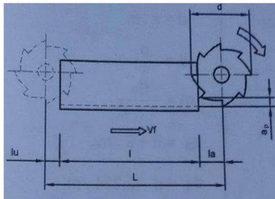
Gambar 2. 6 Gerakan slab milling pada mesin CNC
