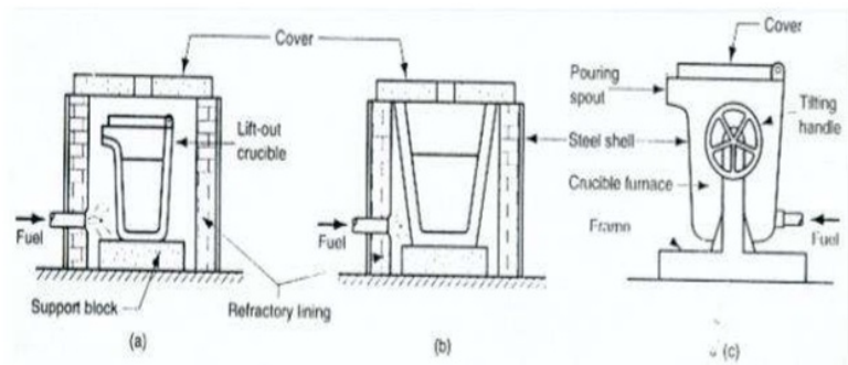
Gambar 2. 16 Tiga Jenis Contoh Dapur Crucible (P.Groover, 2000)
