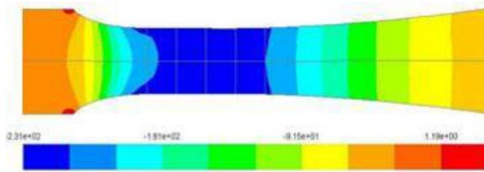
Gambar 5. 3. Distribusi tekanan model RSM untuk U_0 = 6.6 m/s
