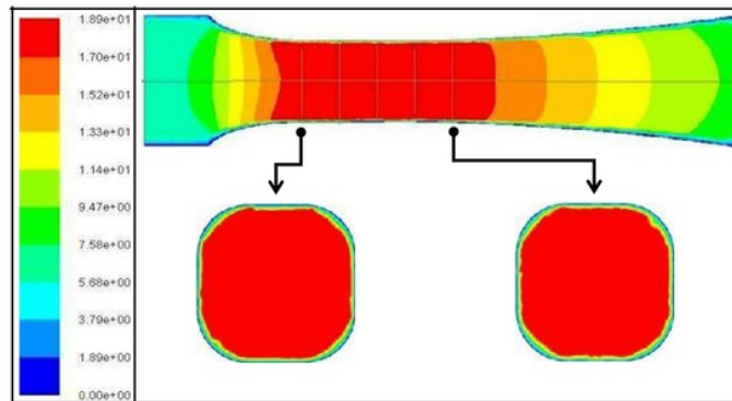
Gambar 5. 2. Distribusi kecepatan model RSM untuk U_0 = 6.6 m/s
