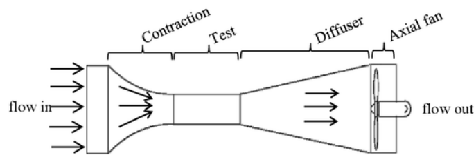
Gambar 2. 2. Terowongan Angin Rangkaian Terbuka tipe suction
