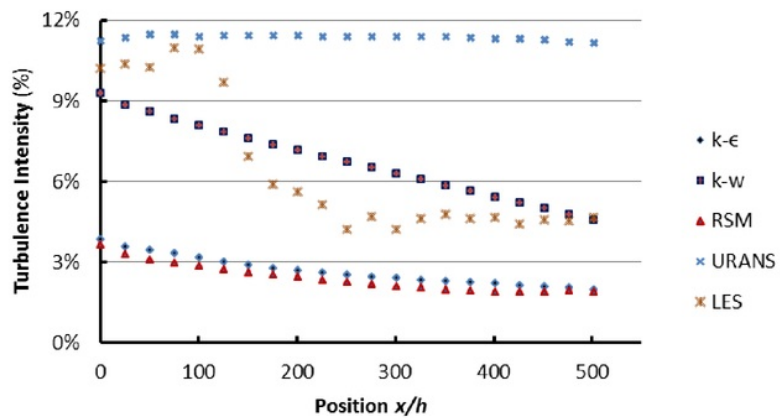
Gambar 5. 4 Turbulence Intensity dari kelima model CFD
