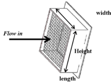
Gambar 2. 4. Settling Section dengan honeycomb
