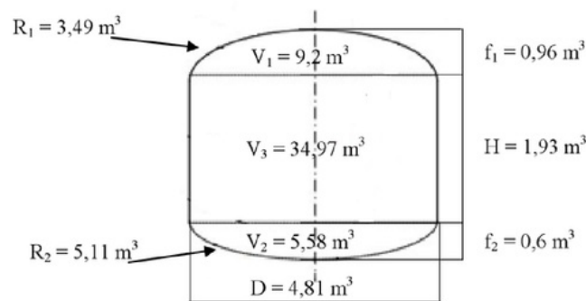
Gambar 2. Hasil Dimensi Reaktor
