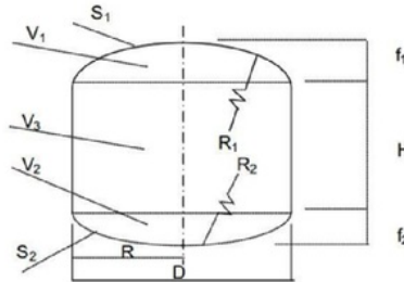
Gambar 1. Dimensi Reaktor[7]
