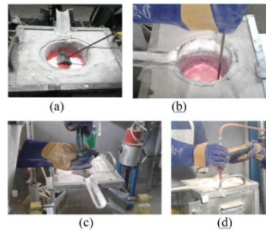
Gambar 3. (a) Proses peleburan (b) Proses degassing menggunakan argon (c) Pemuangan kotoran (d) Proses stirring
