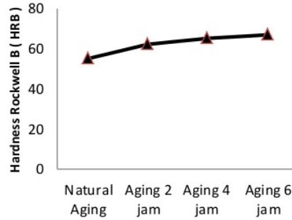
Gambar 11. Grafik hasil pengujian kekerasan untuk temperatur aging 200°C
