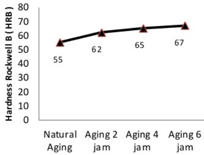
Gambar 9. Grafik hasil pengujian kekerasan untuk temperatur aging 140°C
