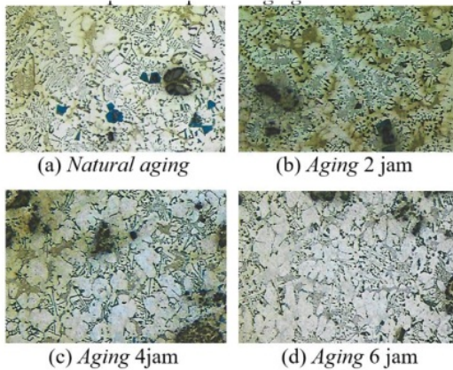
Gambar 13. Struktur mikro aluminium komposit pada temperatur aging 180°C
