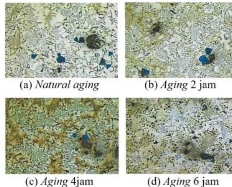
Gambar 12. Struktur mikro aluminium komposit pada temperatur aging 140°C
