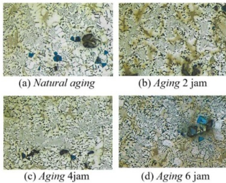
Gambar 14. Struktur mikro aluminium komposit pada temperatur aging 200°C
