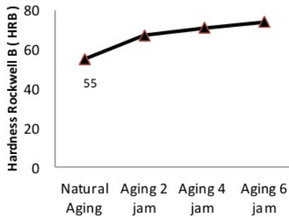
Gambar 10. Grafik hasil pengujian kekerasan untuk temperatur aging 180°C
